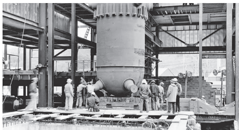
Instalarea unuia dintre primele reactoare nucleare de energie (60 MW). Shippingport NPP, SUA, 1956
